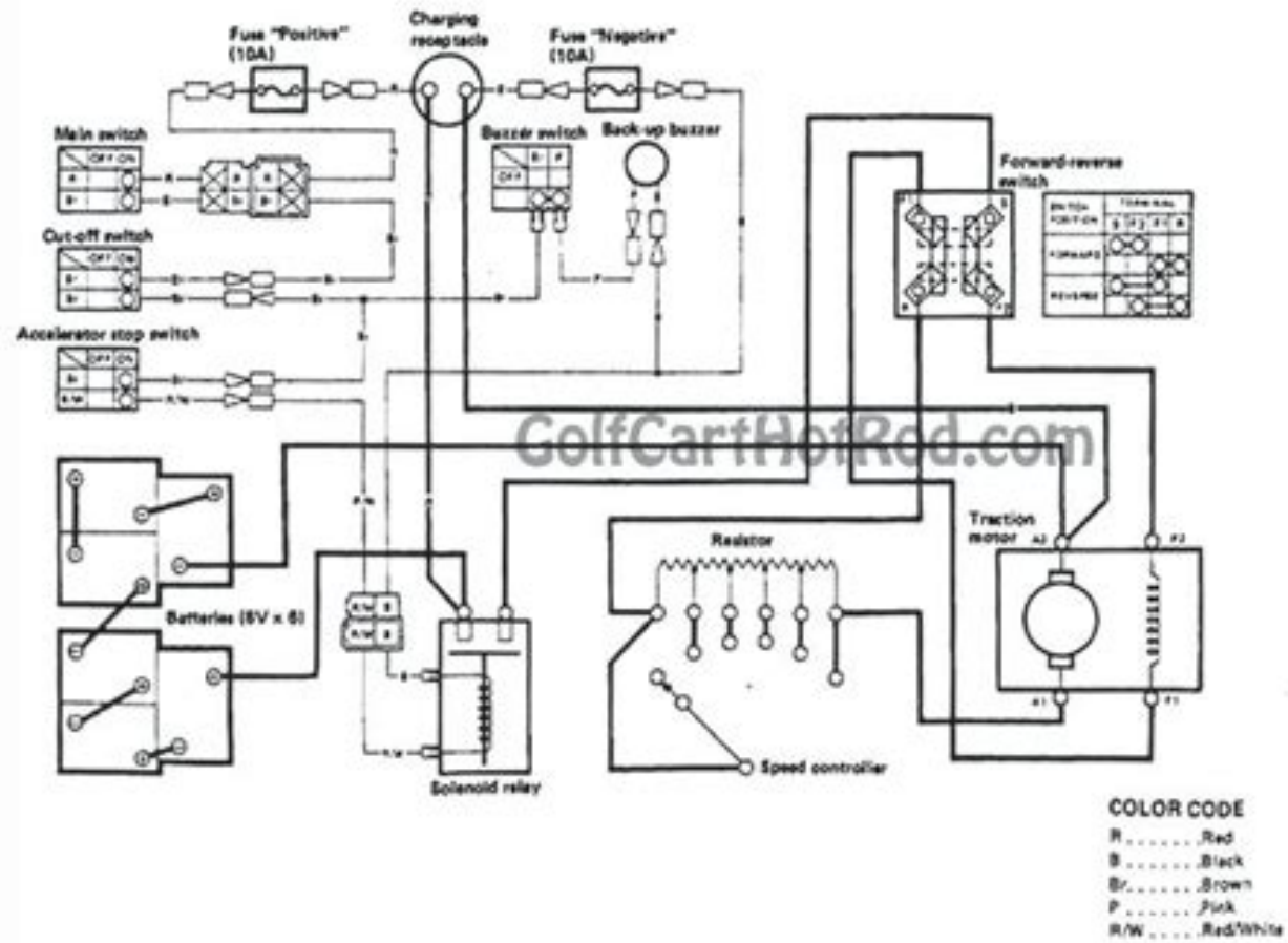
G2E WIRING DIAGRAM
